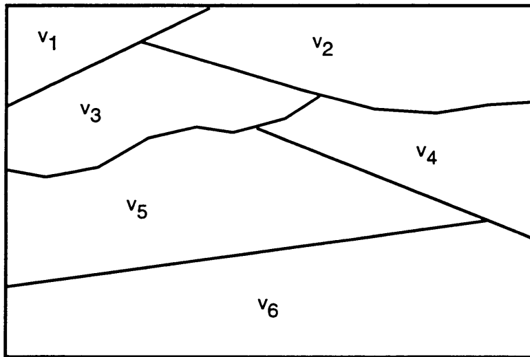
FIG. 5.1. Macro model.
